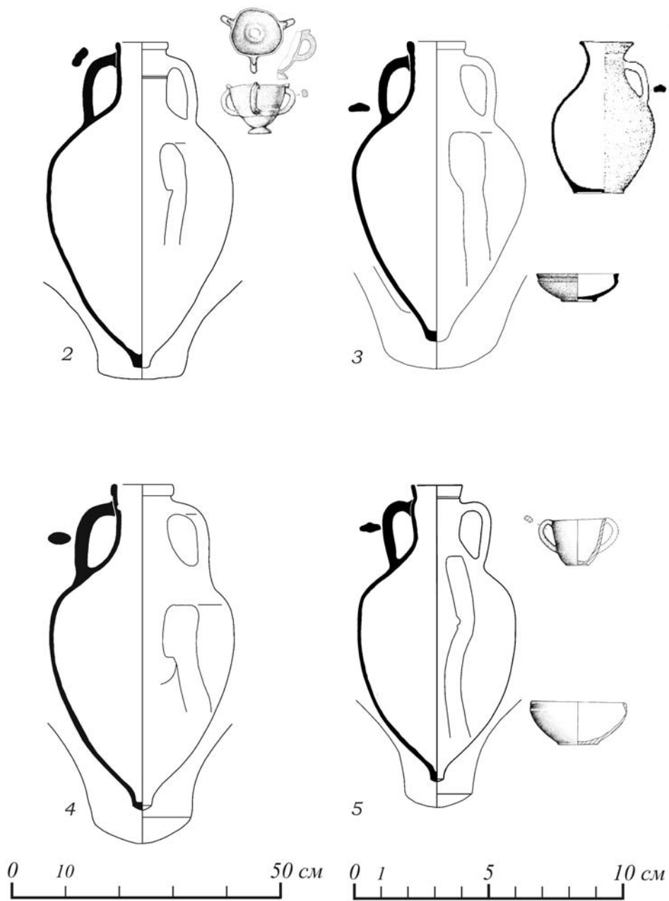
Табл. 2. Амфоры "старокорсунского" типа II (вариант IIА - № 2-5)
